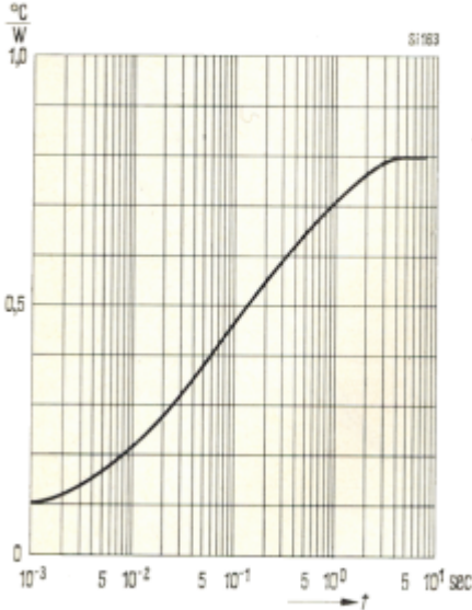
Transienter Wärmewiderstand Z_{th} Freier Aufbau
