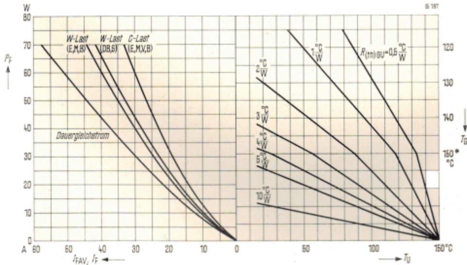
Belastbarkeitsdiagramm
