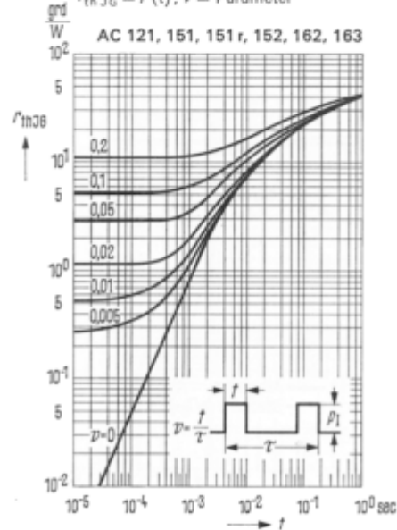
Zulässige Impulsbelastbarkeit r_{\text{thJG}} = f(t) ; v = \text{Parameter}
