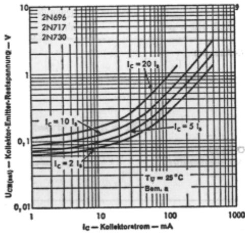
Kollektor-Emitter-Restspannung als Funktion des Kollektorstromes
