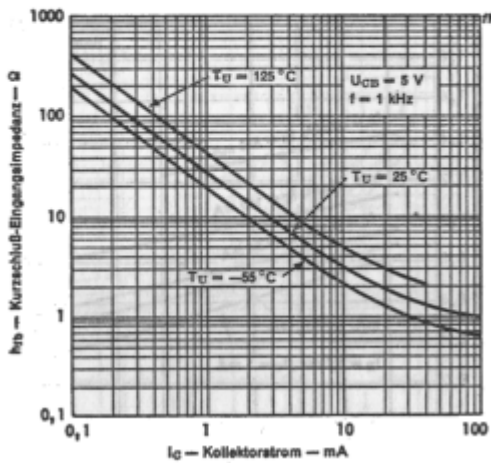
Kurzschluß-Eingangsimpedanz als Funktion des Kollektorstromes
