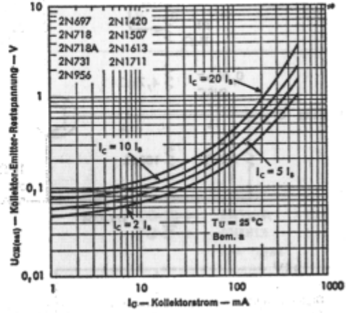
Kollektor-Emitter-Restspannung als Funktion des Kollektorstromes
