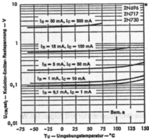
Kollektor-Emitter-Restspannung als Funktion der Umgebungstemperatur
