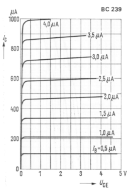
Ausgangskennlinien I_C = f(U_{CE}) : I_B = \text{Parameter (Emitterschaltung)}
