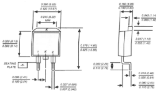
TO-263AB
